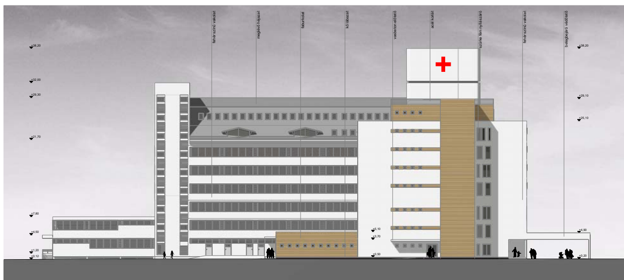
ÉSZAKKELETI HOMLOKZAT M=1:200
