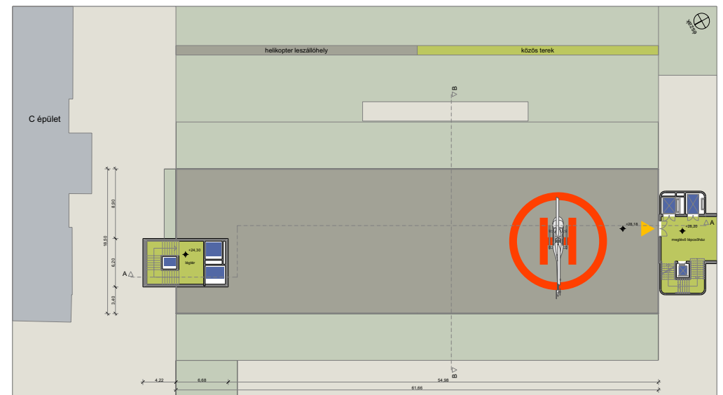
TETŐSZINTI ALAPRAJZ M=1:200
