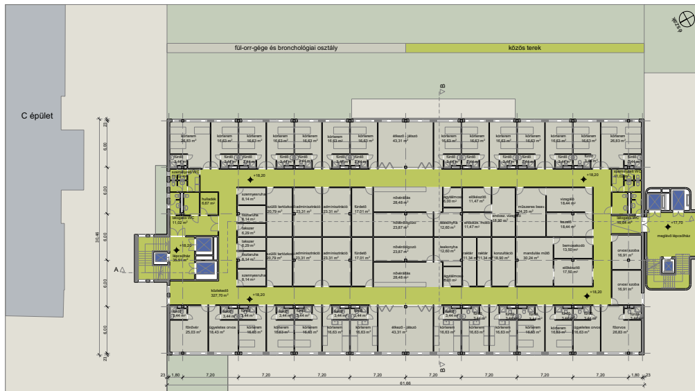
5. EMELETI ALAPRAJZ M=1:200
