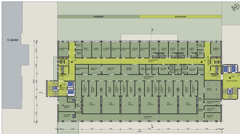
2. EMELETI ALAPRAJZ M=1:200
