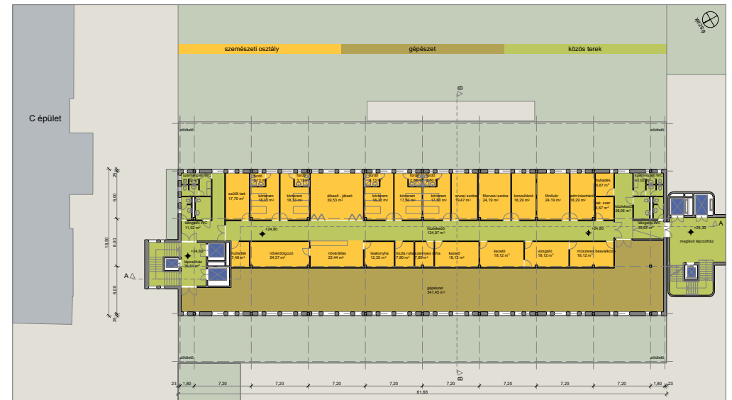
7. EMELETI ALAPRAJZ M=1:200
