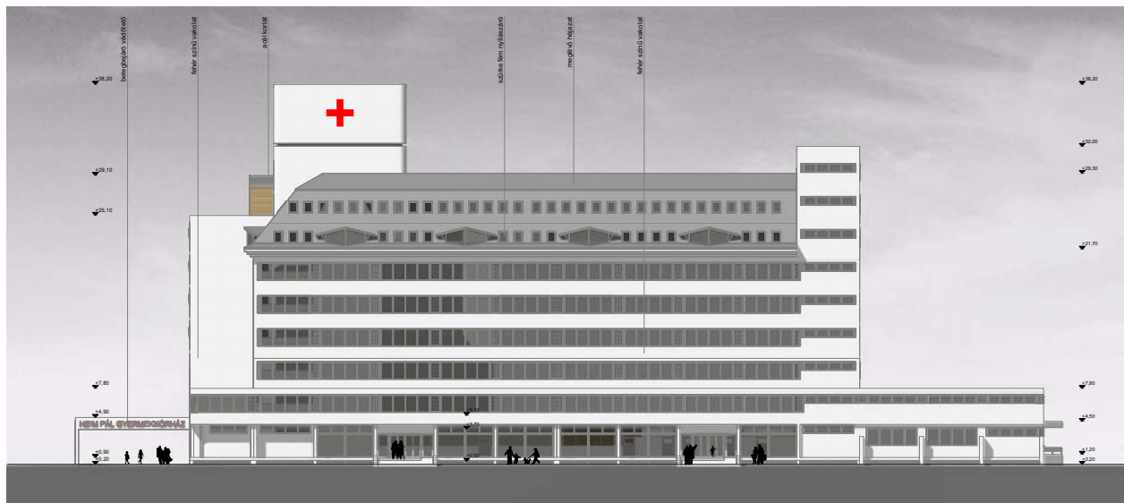
DÉLNYUGATI HOMLOKZAT M=1:200
