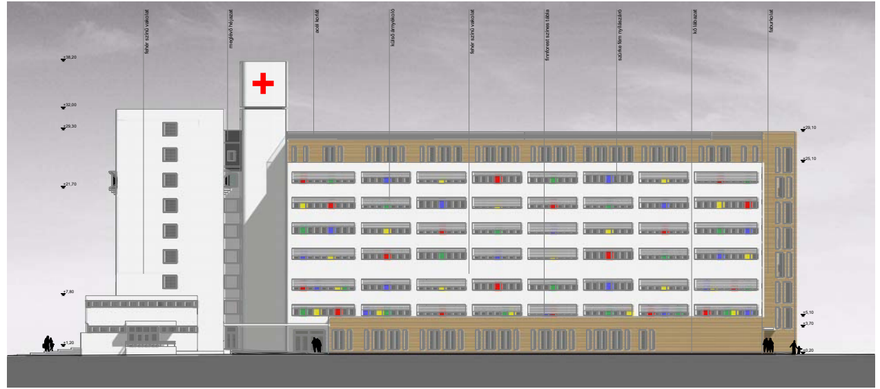
DÉLKELETI HOMLOKZAT M=1:200
