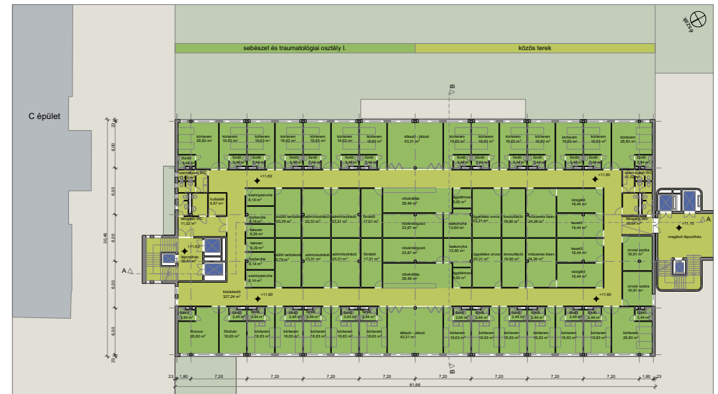
3. EMELETI ALAPRAJZ M=1:200
