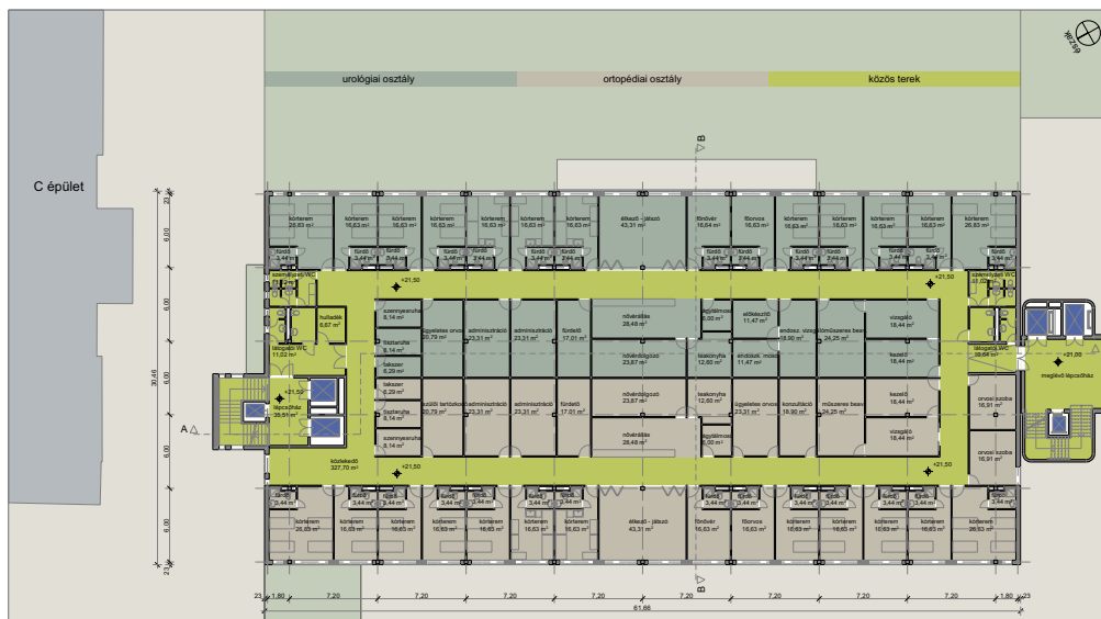
6. EMELETI ALAPRAJZ M=1:200
